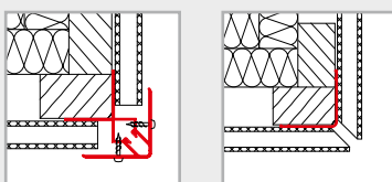
Buitenhoek C
