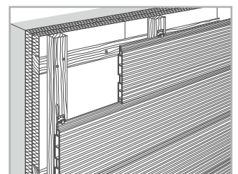
Voorbeeld horizontale montage van structura, profielkant linea.
