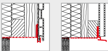
Beginprofiel P
