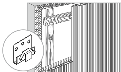
Voorbeeld verticale montage van structura, profielkant banda.
