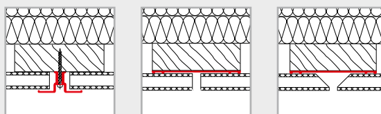
Afdekprofiel
